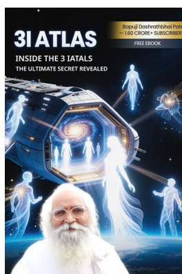
3i Atlas
